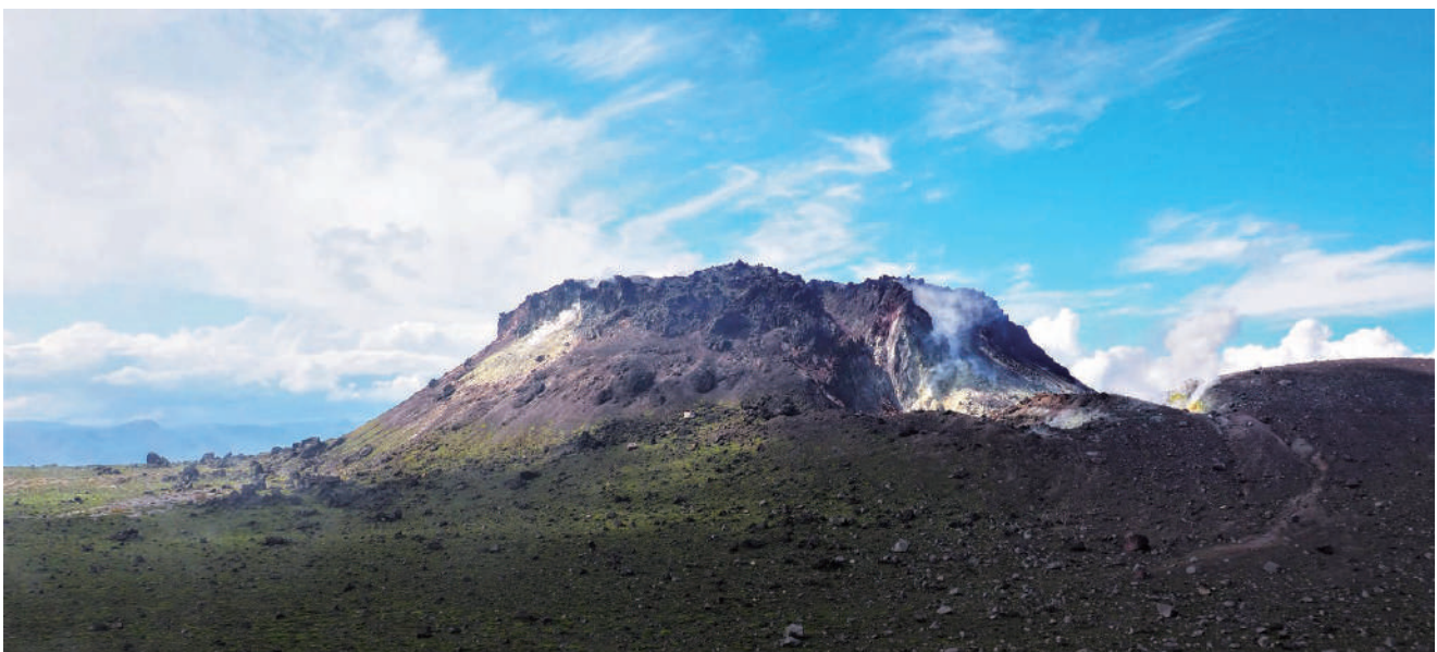
樽前山
